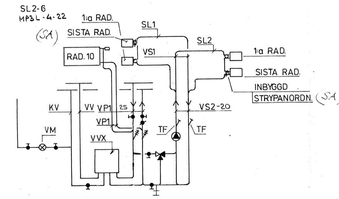
DETALJ INKOPPLING AV VVX
